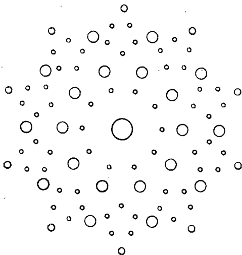
Рис. 21. Квазикристаллический спектр
