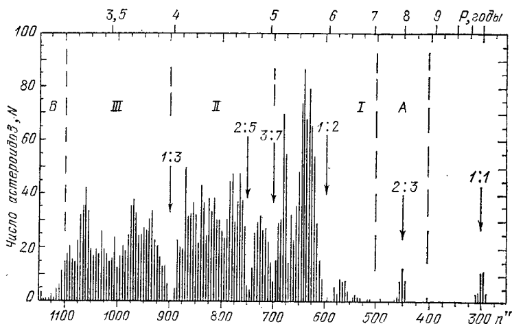
Рис. 24. Люки Кирквуда
