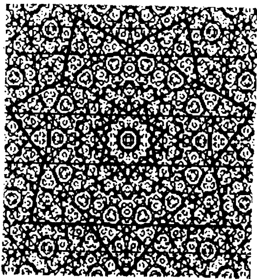
Рис. 41. Стохастическая паутина
