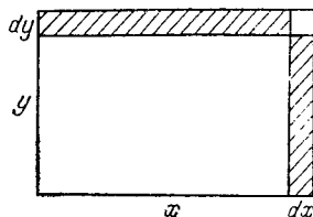
Рис. 9. Формула Лейбница
