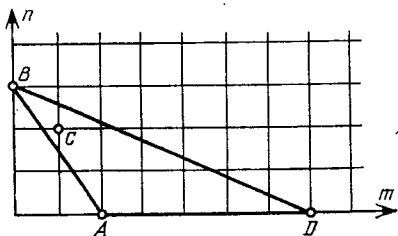
Рис. 7. Многоугольник Ньютона
